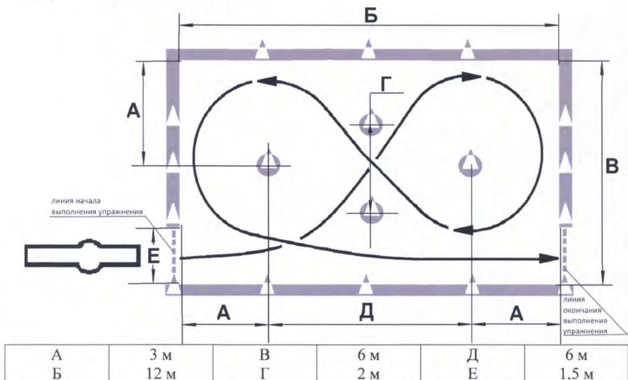
Рисунок 4. Схема и размеры элемента упражнения № 1 - «Габаритная восьмерка»
