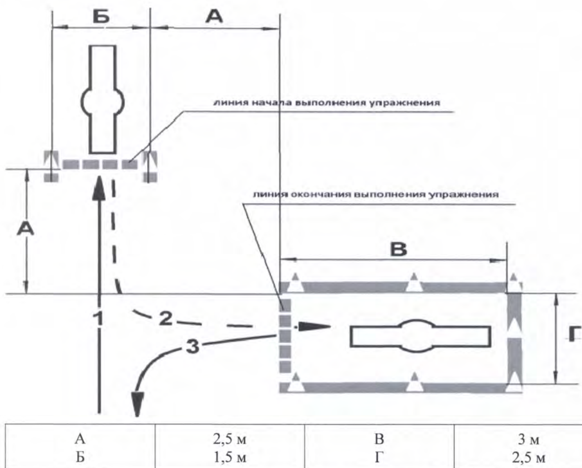
Рисунок 5. Схема и размеры упражнения № 2
