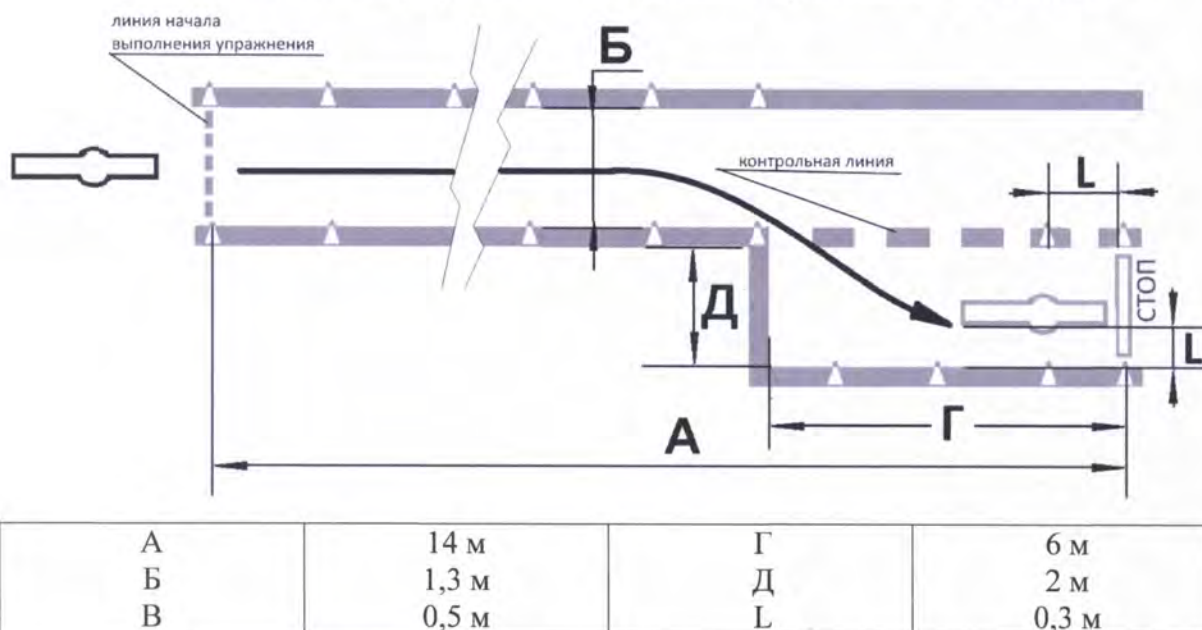
Рисунок 6. Схема и размеры упражнения № 3
