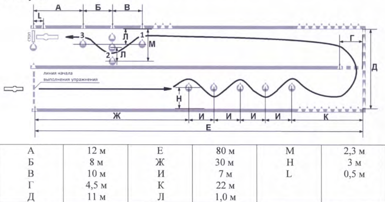
Рисунок 3. Схема и размеры элемента упражнения № 1 – «Скоростное маневрирование»
